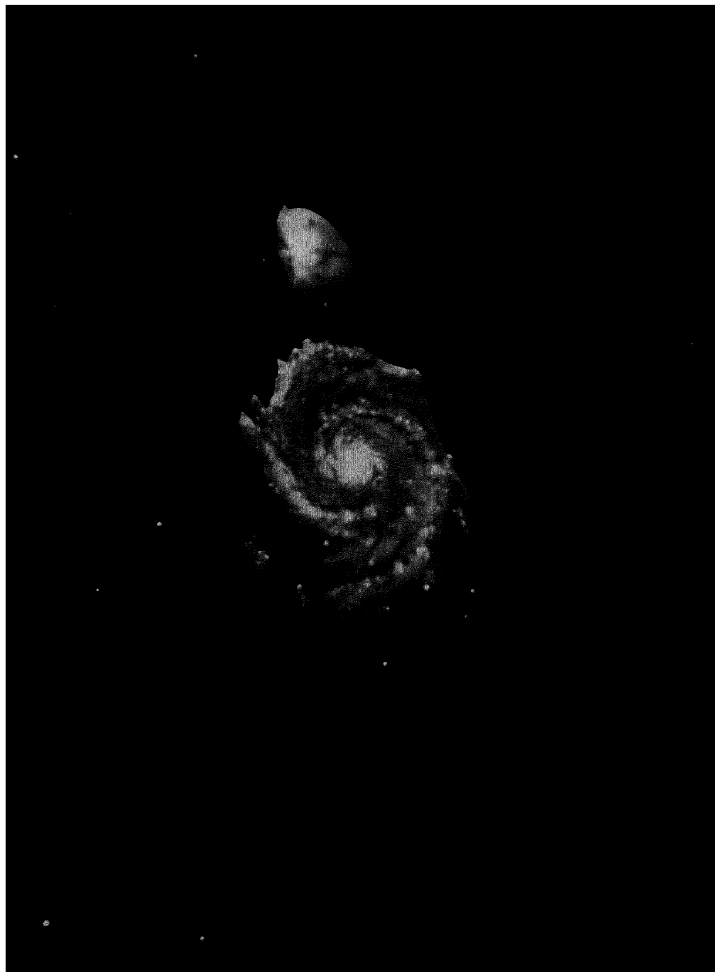
SPIRAL NEBULA M. 51 in Canes Venatici
